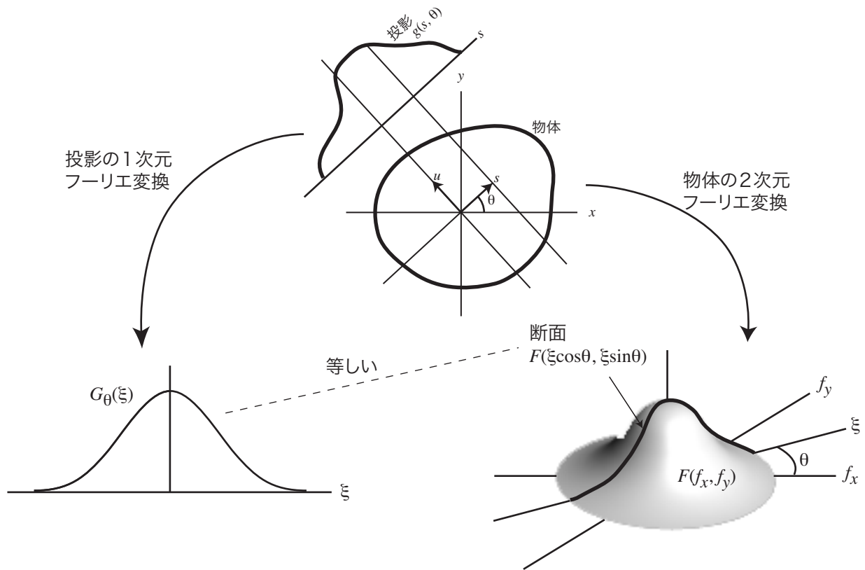
図 3: 投影定理.
