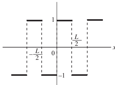
図 2: 例題の関数.
