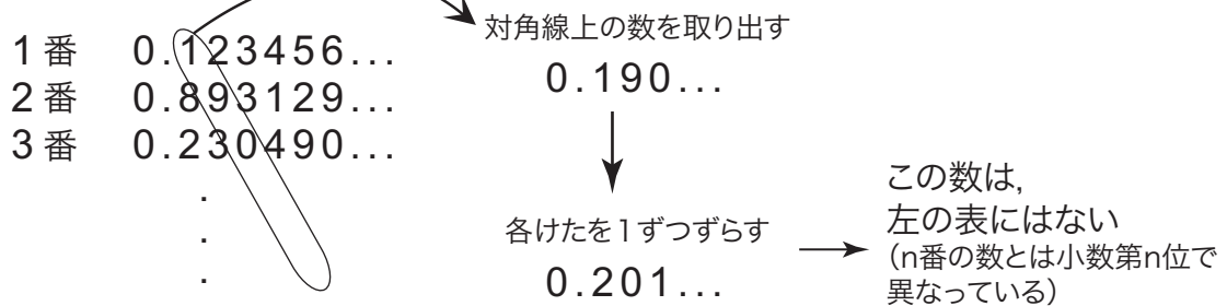
図 2: 対角線論法
