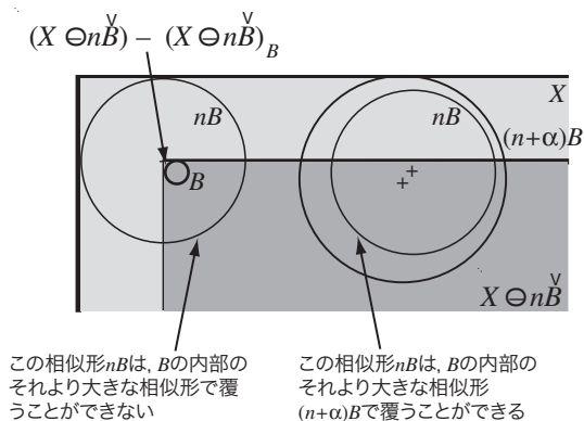
図 3: (8) 式の意味
