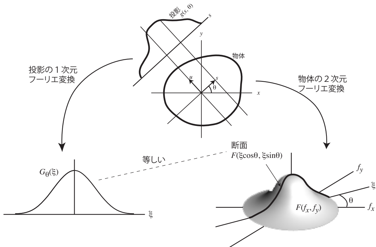
図 3: 投影定理.
