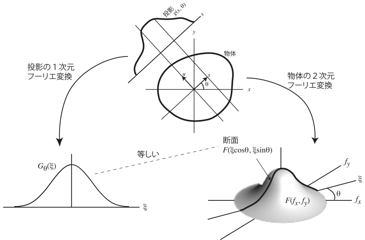
図 1: 投影定理.
