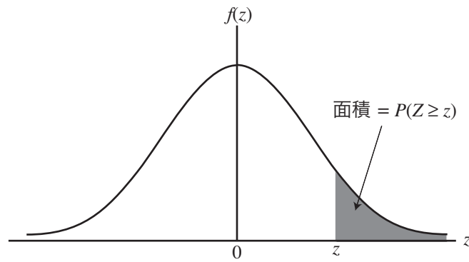
図 5: 標準正規分布の確率密度関数のグラフ上で「確率変数 Z が値 z 以上である確率」 P(Z \geq z)
