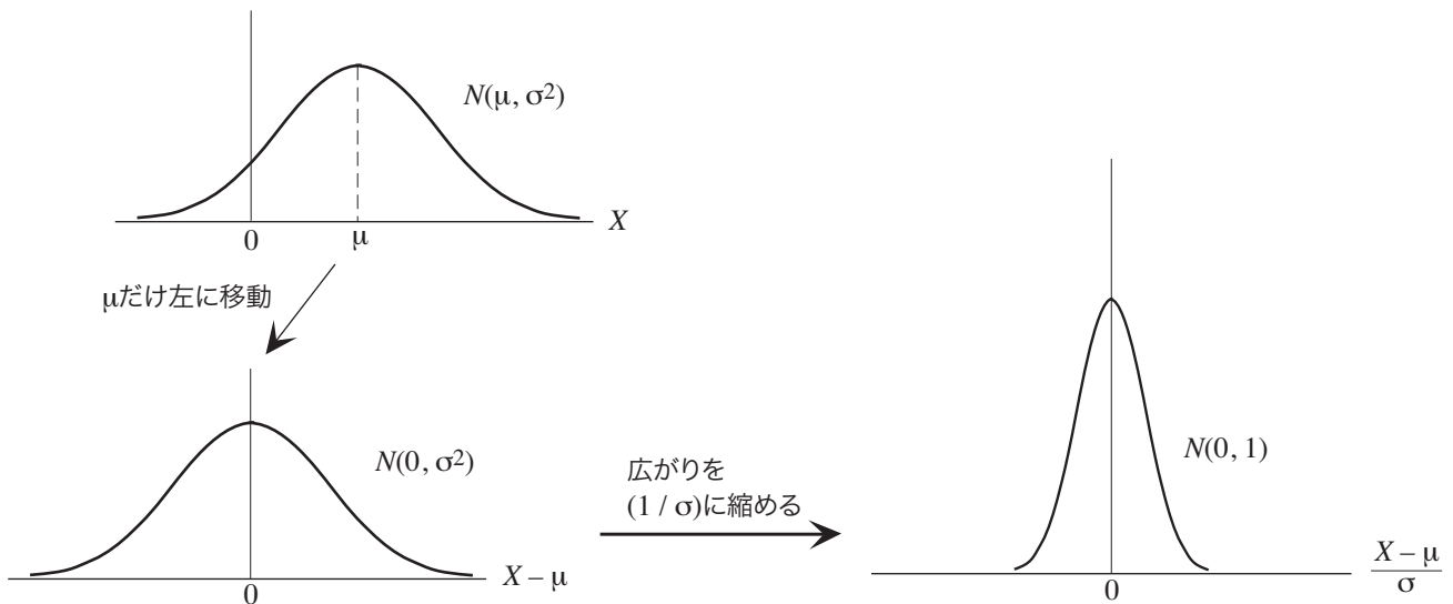
図 4: 正規分布の性質 1
