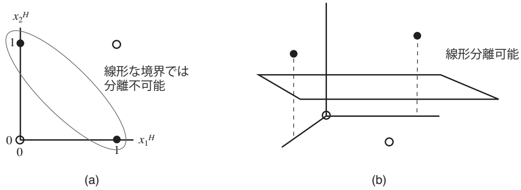
図 10: 高次元空間への変換
