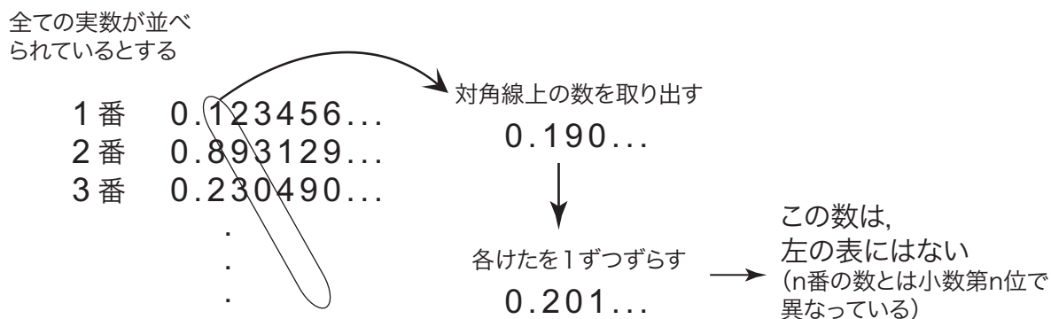
図 2: 対角線論法
