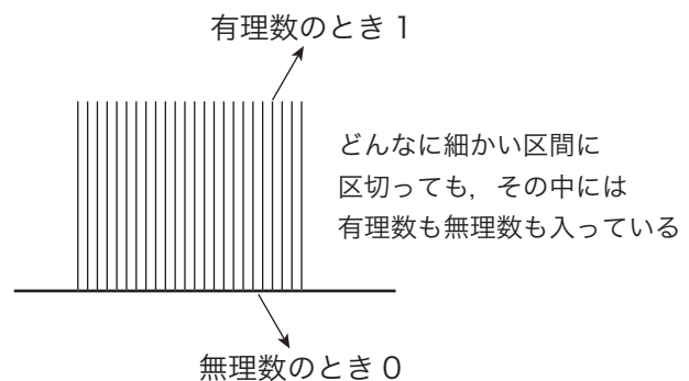
図 2: ディリクレ関数の積分
