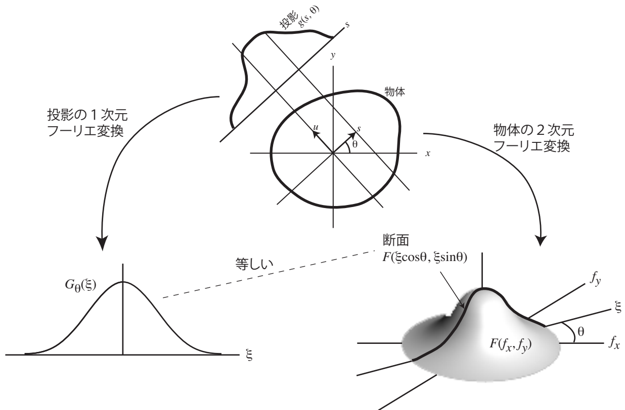
図 3: 投影定理.
