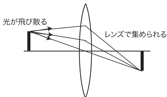
図 1: 結像.
