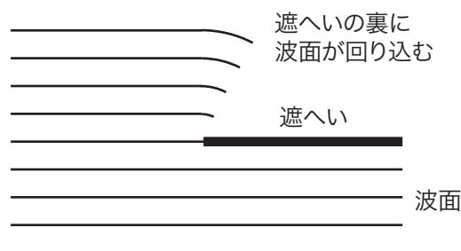
図 2: 回折.
