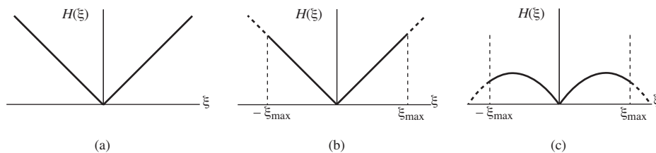
図 2: 種々のフィルタ関数. (a) オリジナルのフィルタ関数 ( |ξ| ). (b) Ram-Lak フィルタ. (c) Shepp-Logan フィルタ.
