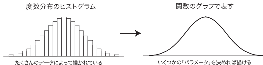
図 1: 確率分布モデル
